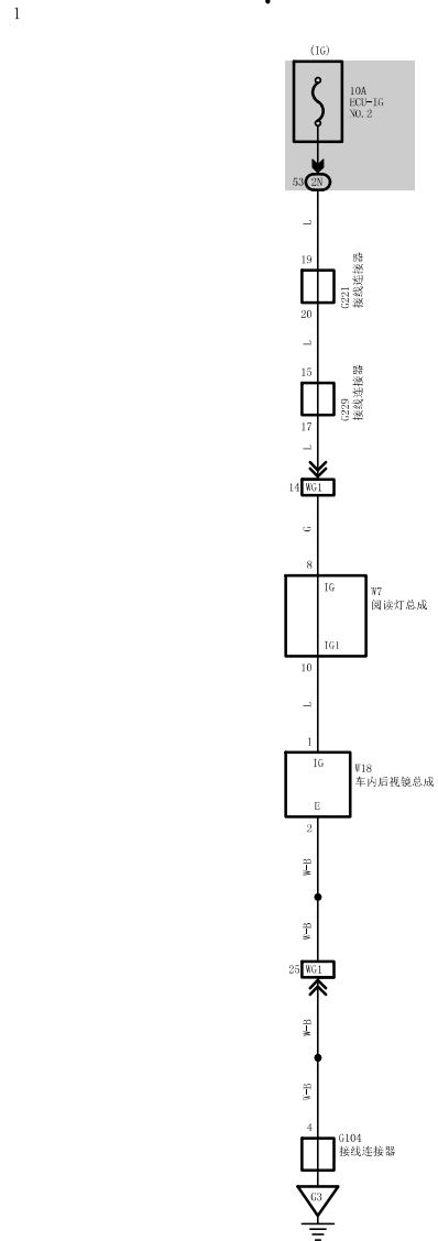
自动防眩目 EC 后视镜 (2017 年 10 月之后生产)
