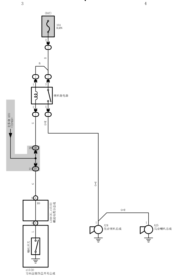
喇叭 (2017 年 10 月之后生产)
